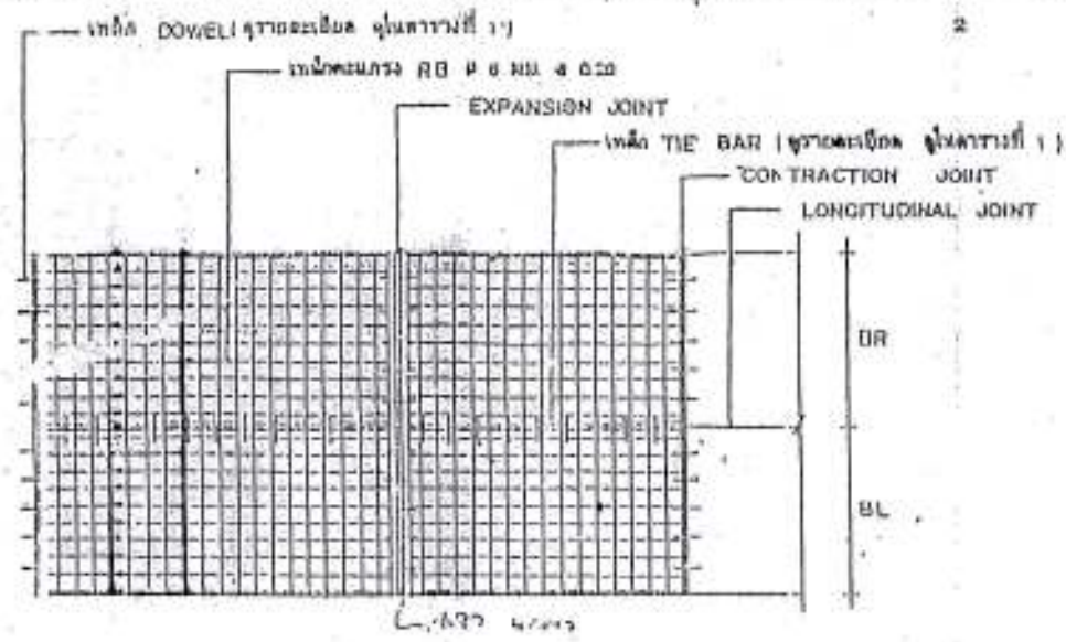
แปลนการวางคานระงเหล็ก
