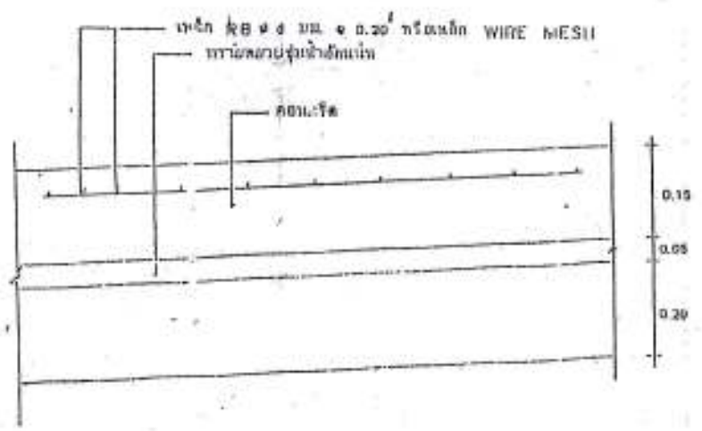
รายละเอียดของถนนคอนกรีตเสริมเหล็ก
